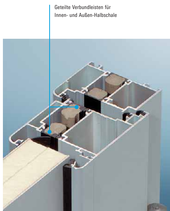
Profilkontur Royal S 75SL.HI innen aufschlagend, außen Softlinekontur
