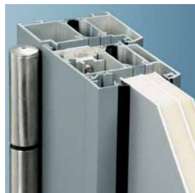
Sicherheits-Türfüllung mit 1,5 mm Aluminiumkern
