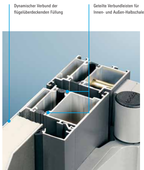
Profilkontur Royal S 70 mit flügelüberdeckender Füllung, innen flächenbündig
