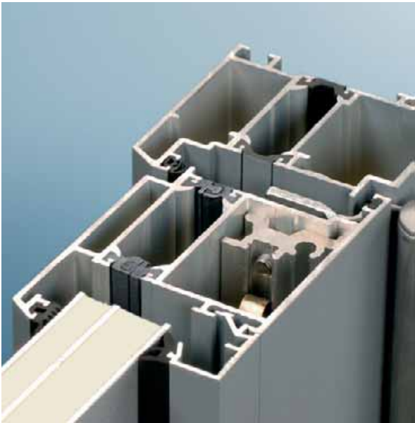
Profilkontur Royal S 65AK innen flächenbündig, außen Althauskontur
