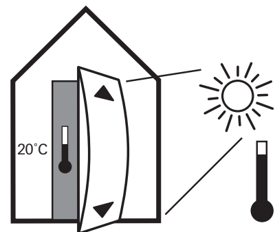
Der Bi-Metall-Effekt bei Türen ohne spannungsfreien Verbund
