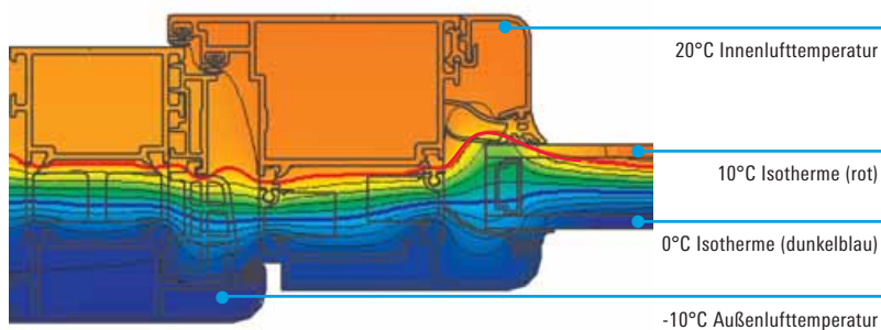
Wärmedämmung der Schüco Haustür
